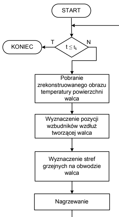
Rys. 2. Schemat ogólny regulacji dwuwymiarowego pola temperatury
