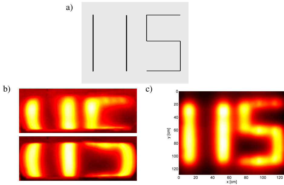
Rys. 7. Wartość zadana temperatury powierzchni walca (a), przykładowe obrazy otrzymane z kamery termowizyjnej (b) oraz uzyskany rozkład temperatury (c)
