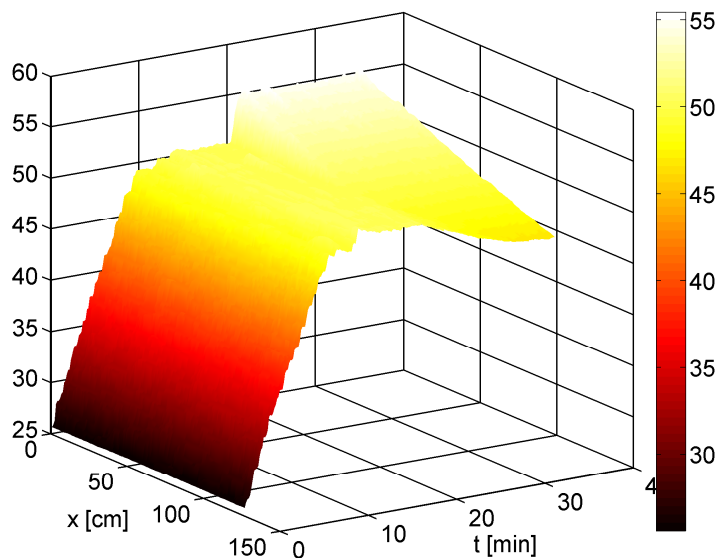
Rys. 5. Rozkład temperatury wzdłuż tworzącej walca w czasie
