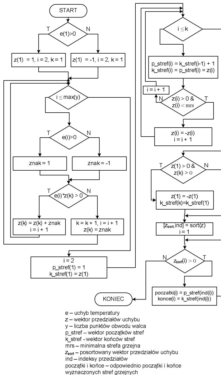
Rys. 4. Sieć działań algorytmu wyznaczania stref grzejących wzdłuż obwodu walca
