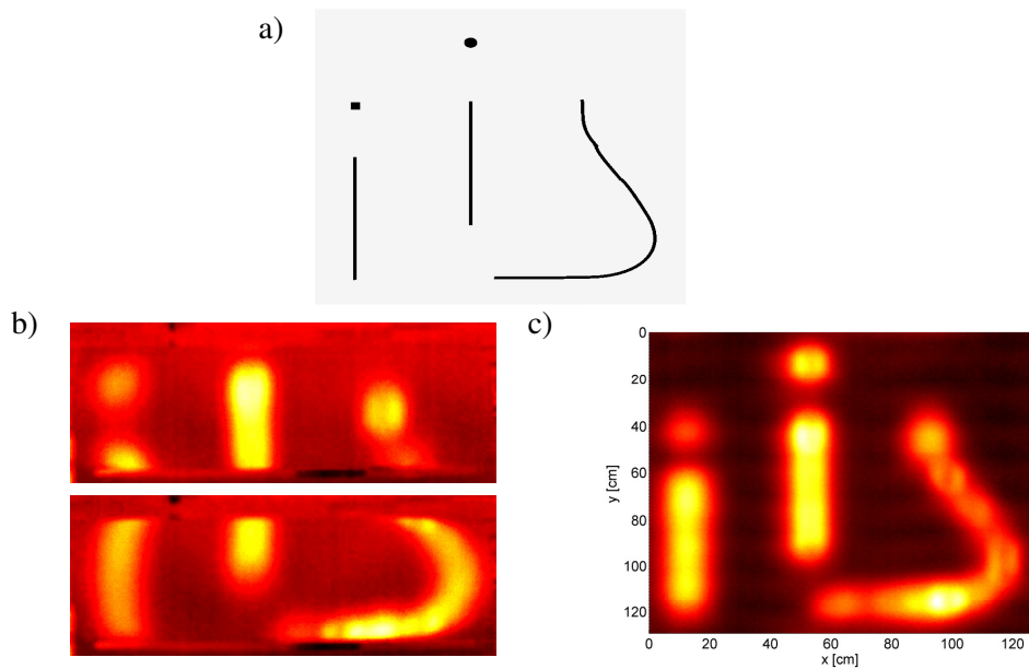
Rys. 8. Wartość zadana temperatury powierzchni walca (a), przykładowe obrazy otrzymane z kamery termowizyjnej (b) oraz uzyskany rozkład temperatury (c)
