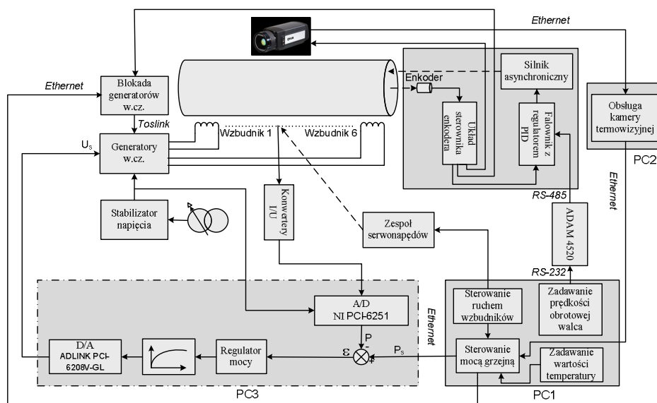
Rys. 1. Schemat stanowiska badawczego
