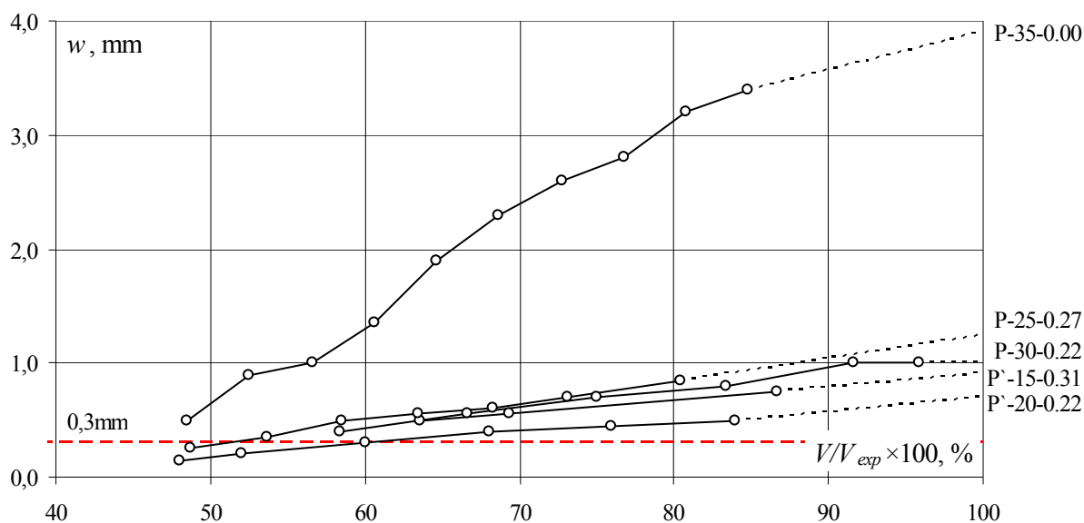
Rys. 3.27. Porównanie rys o maksymalnej szerokości rozwarcia modeli serii trzeciej w zależności wyężenia elementów Fig. 3.27. Comparison of the cracks of maximum width of third series models in relation to the elements effort
