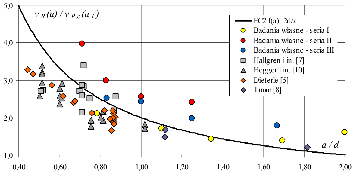
Rys. 4.1. Wartości stosunku v_{exp}(u)/v_{R,c}(u_1) w zależności od smukłości ścinania a/d – badania własne i obce Fig. 4.1. Values of the ratio v_{exp}(u)/v_{R,c}(u_1) in relation of the shear slenderness a/d – own and other investigations
