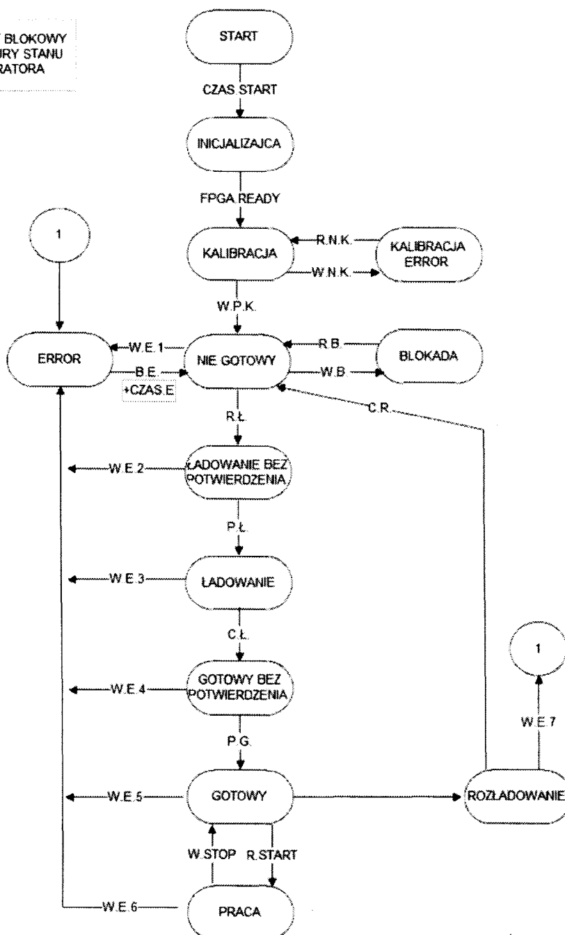
Rys. 2. Schemat blokowy algorytmu stanu w prototypowym generatorze
