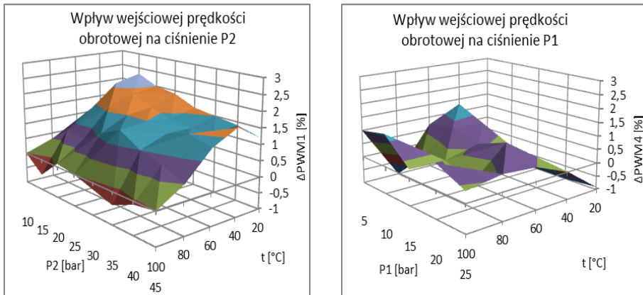
Rys. 8. Zestawienie map przedstawiające różnice w sygnałach PWM potrzebne do uzyskania tego samego ciśnienia P2 lub P1 pomiędzy skrajnymi wejściowymi prędkościami obrotowymi
