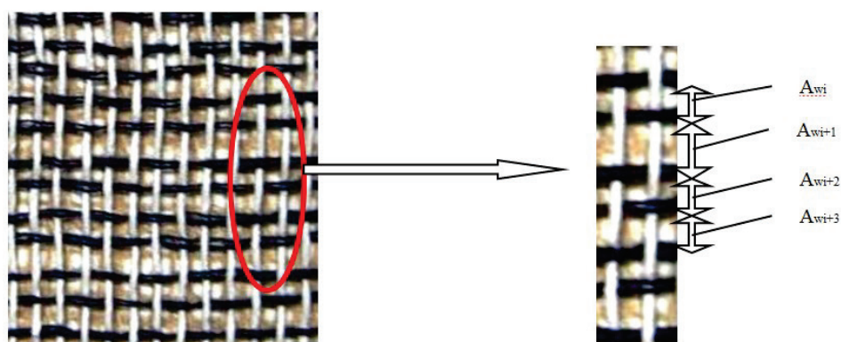
Rys. 11. Metoda pomiaru podziałki wątku
