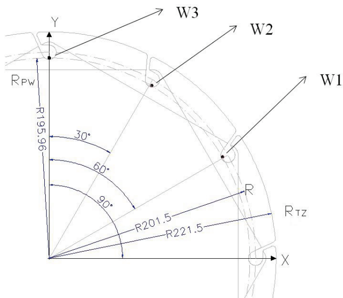
Rys. 6. Schemat wycinka wału tkającego zastosowany w analizie
